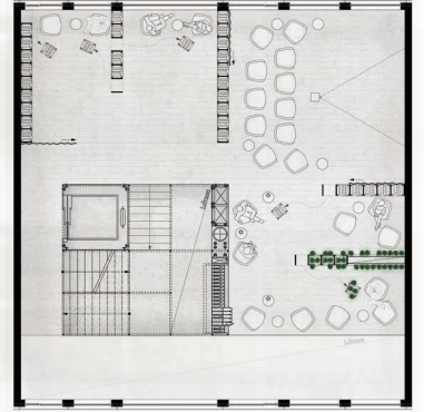
5. OBERGESCHOSS M1.50
