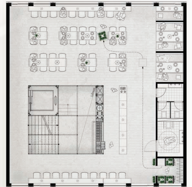
1. OBERGESCHOSS M1.50
